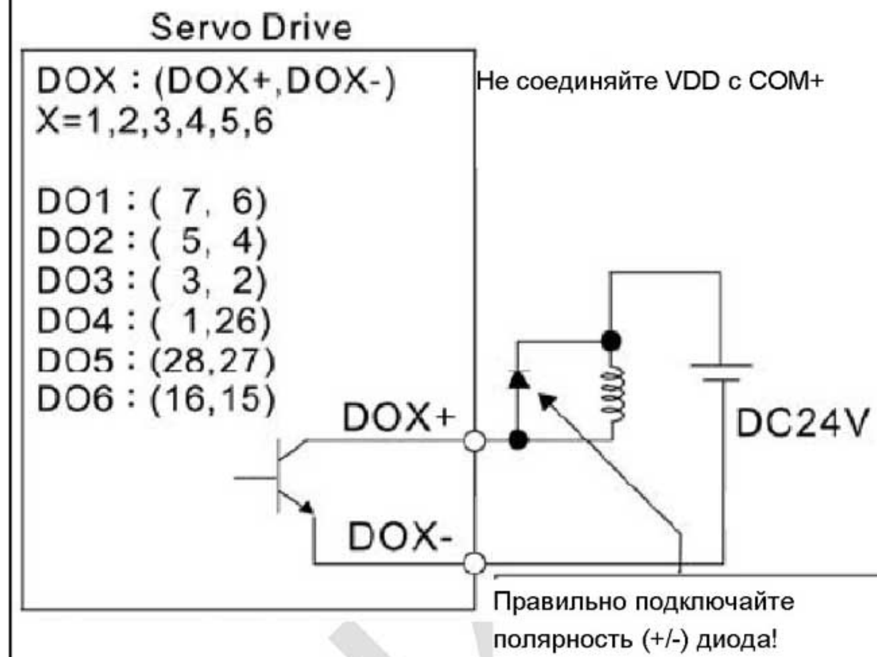
C8: Подключение выходных сигналов (DO) при использовании внешнего источника питания для индуктивной нагрузки
