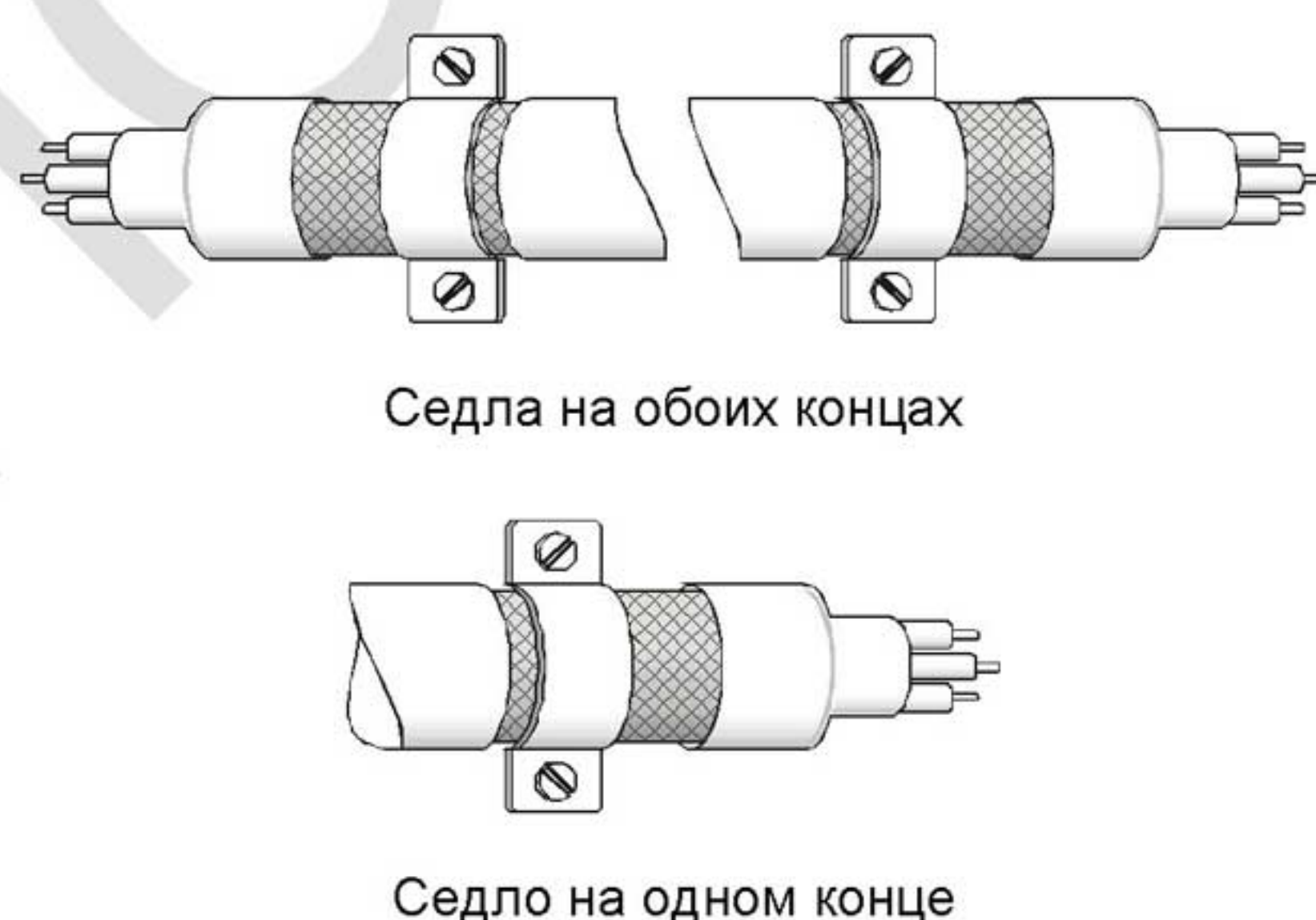
Рисунок 2. Соединение экрана с двух сторон кабеля
